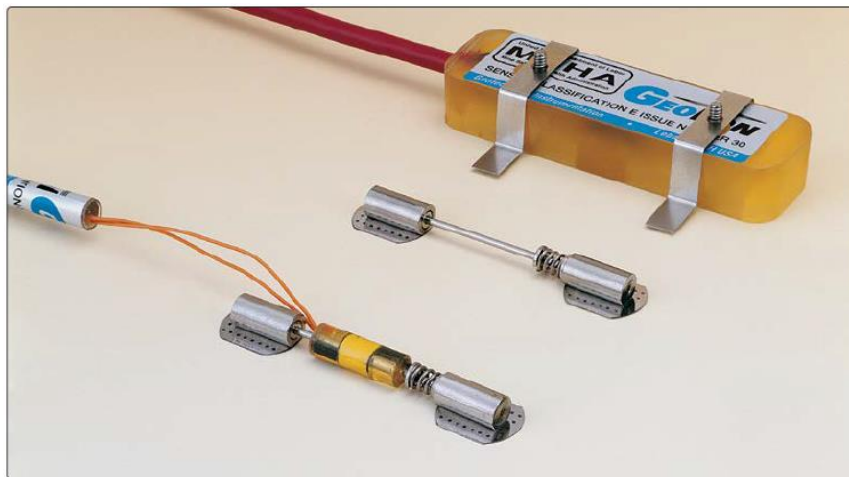
El Modelo 4150 (al frente) y Deformímetro soldable de punto Modelo 4100
